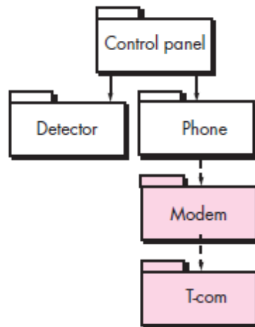
Fig 10.5: Layer cohesion
